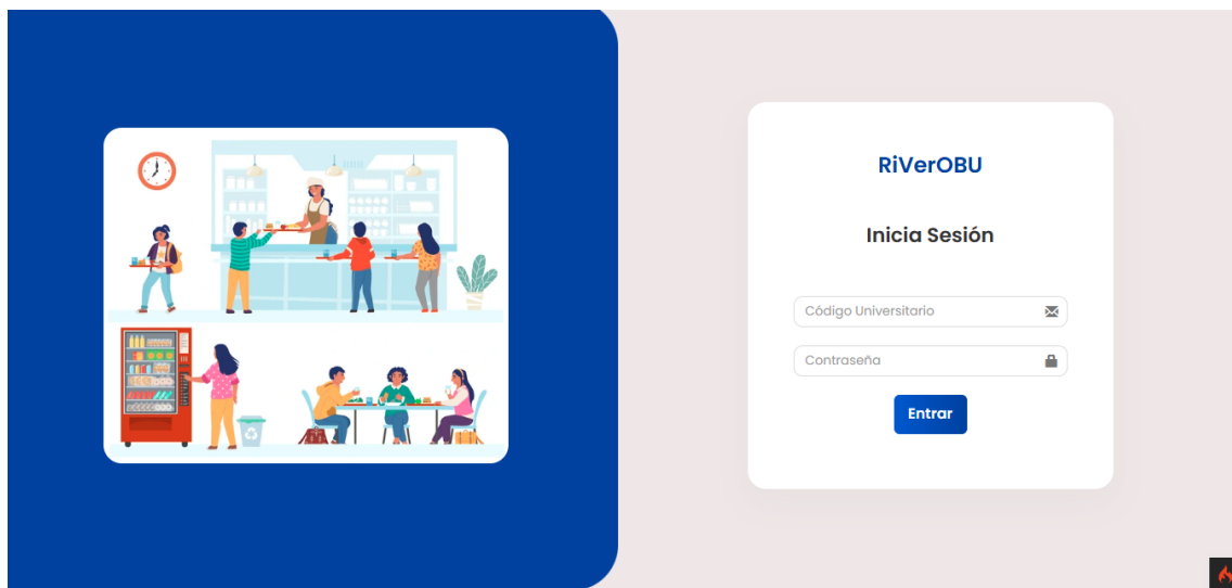
Figura 1. Login Administrador
